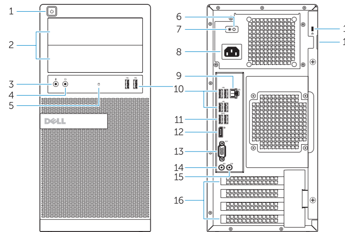
OptiPlex 3020 MT
